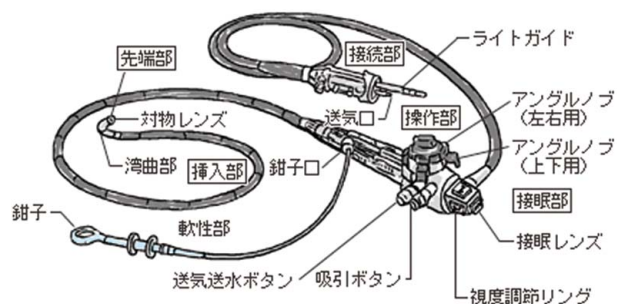
【図1】 内視鏡の構造
